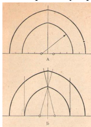
2-расм. Исмоил Сомоний мақбарасидаги икки марказ орқали ясаладиган равоқ
