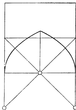
5-расм. Улуғбек мадрасасидаги уч марказ орқали ясаладиган равоқ
