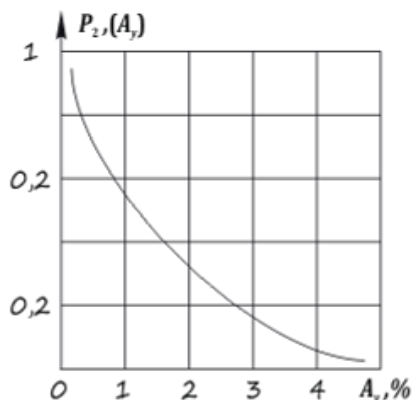
Рис. 3. График распределения вероятности снижения полноты сбора хлопкоуборочных аппаратов при поперечных колебаниях уборочных аппаратов.
