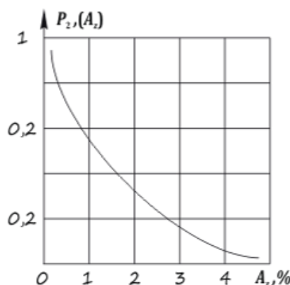
Рис. 4. График распределения вероятности снижения полноты сбора хлопкоуборочных аппаратов при вертикальных колебаниях уборочных аппаратов.
